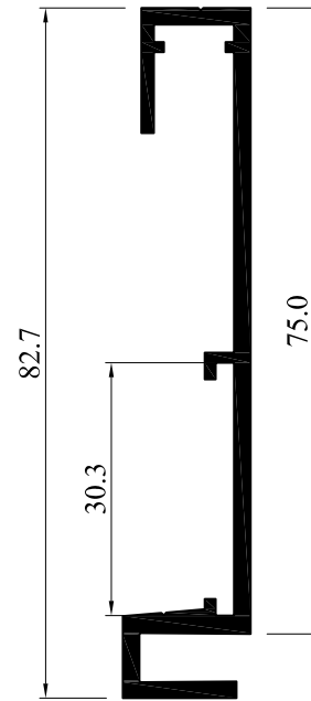
54050-20 Alüminyum Ahşap ve Cam Kapı Ek Profili
