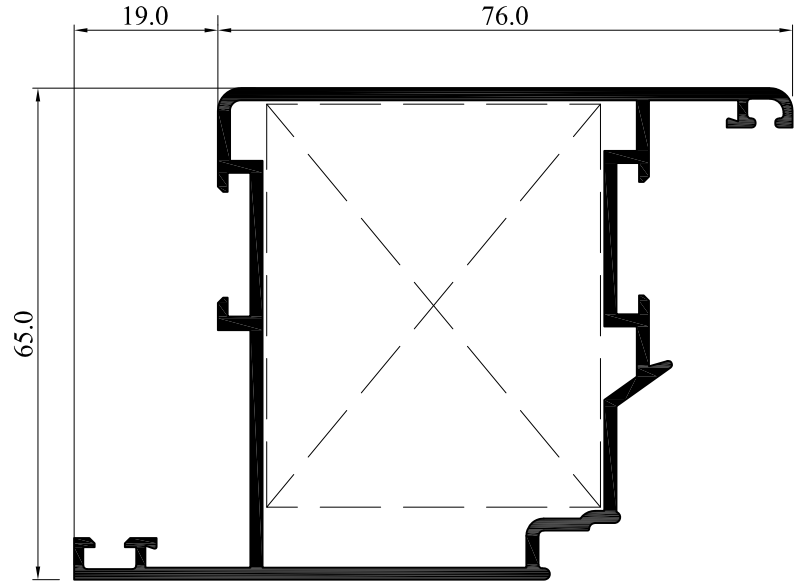
12382-16 Sistem Kapı Profili
