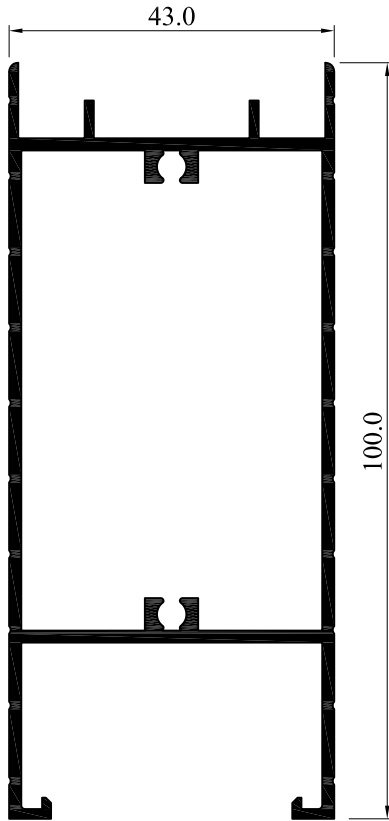
54111-16 Ahşap ve Cam Etek Profili
