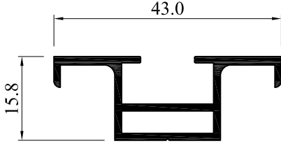
54112-16 Cam Kapı Etek İlave Profili
