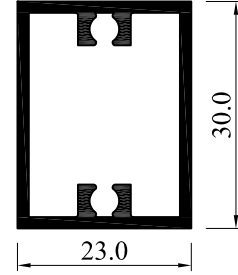
54021-15 Ahşap Kapı Orta kayıt Profili
