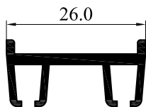
1269-00 Etek Fırçalık Profili
