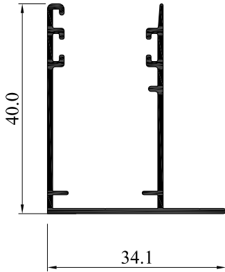
9480 0.359 Kg/m
