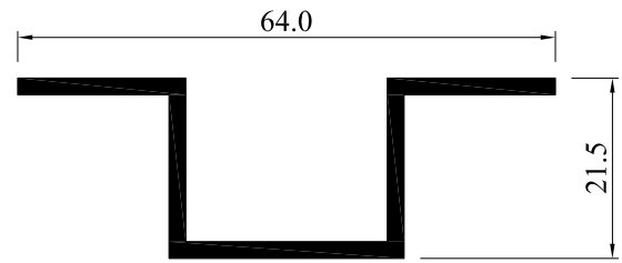
5779-20 0.558 Kg/m
