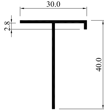
5788-12 5788-30 0.233 Kg/m 0.567 Kg/m
