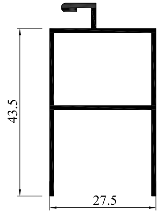
596 0.469 Kg/m
