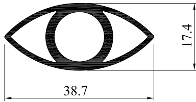
9307 0.512 Kg/m
