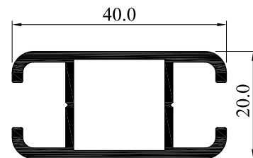
9001 0.570 Kg/m
