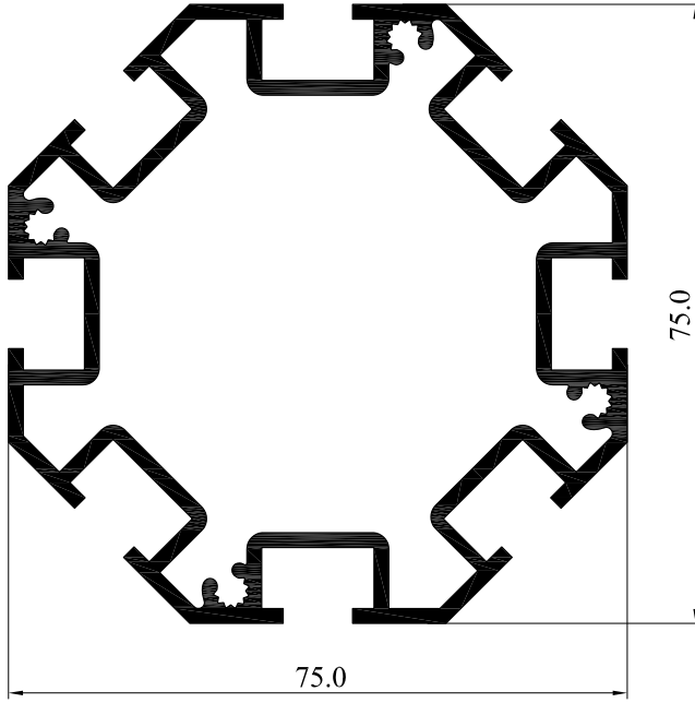
629 2.176 Kg/m
