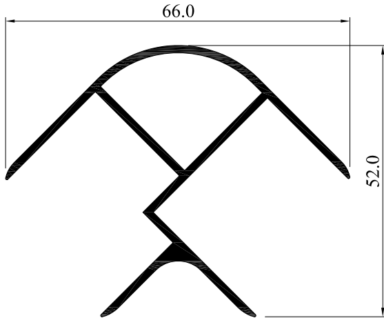
9425 1.028 Kg/m
