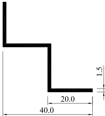
186 0.319 Kg/m
