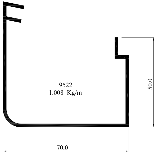
ATM Reklam Panosu Işıklandırma Profili
