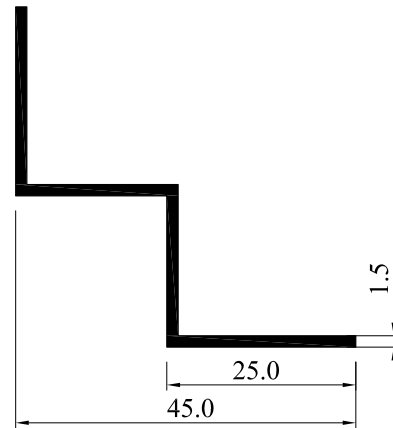
187 0.360 Kg/m
