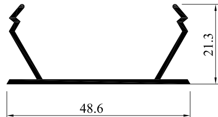
5305-12 0.310 Kg/m
