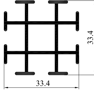
1053 0.655 Kg/m
