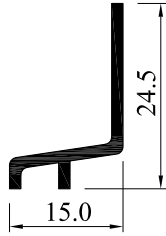
5782-15 0.155 Kg/m
