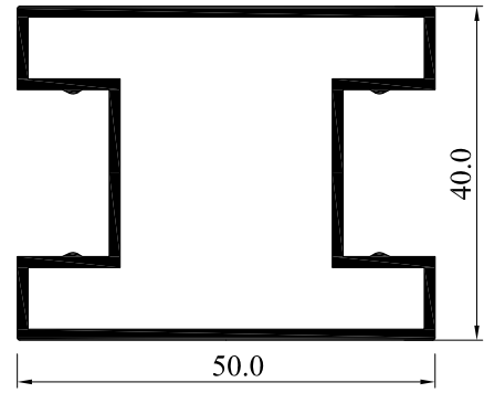
988 0.778 Kg/m
