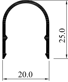
5310-12 0.201 Kg/m
