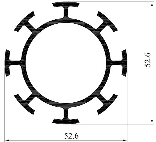
9002 1.211 Kg/m
