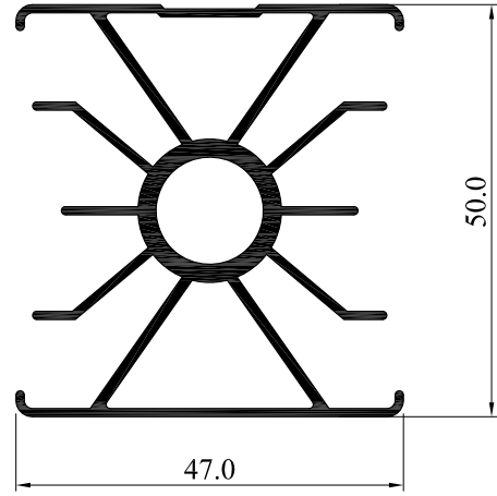
9304 1.041 Kg/m
