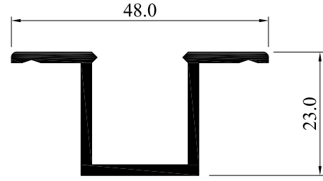
5778-20 0.489 Kg/m
