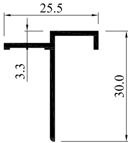
5784-12 0.193 Kg/m
