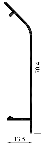
57771-12 0.301 Kg/m
