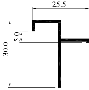
5793-12 0.191 Kg/m
