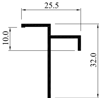
5783-12 5783-15 0.214 Kg/m 0.266 Kg/m 5783-20 0.353 Kg/m
