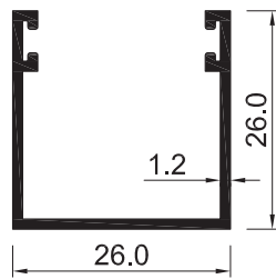
5506-12 0.282 kg/m
