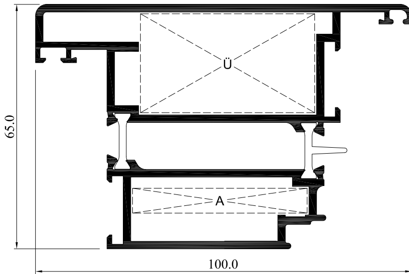
DIŞA AÇILIR KAPI KANAT PROFİLİ
