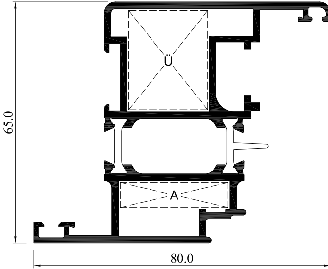
PVC AKSESUAR İÇİN KANAT
