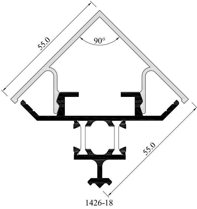
90° AÇI İÇİN
