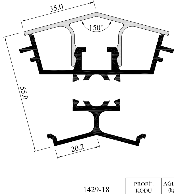
150° AÇI İÇİN
