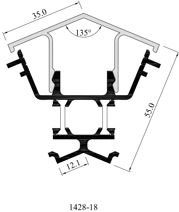
135° AÇI İÇİN
