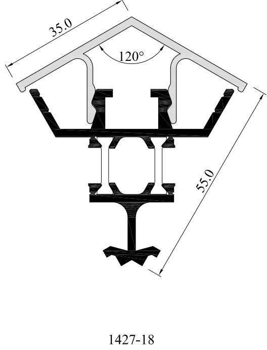
120° AÇI İÇİN
