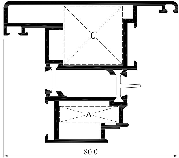
DIŞA AÇILIR KAPI KANAT PROFİLİ
