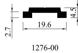
TİJ PROFİLİ
