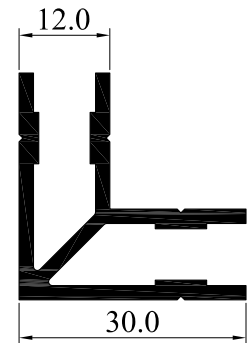
3181-00 0.601 Kg/m
