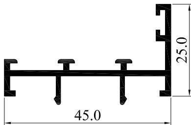
3150-15 0.451 Kg/m
