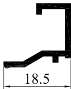
32631-15 0.179 Kg/m
