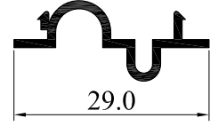
3152-12 0.169 Kg/m
