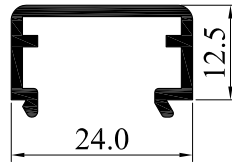
3138-15 0.241 Kg/m
