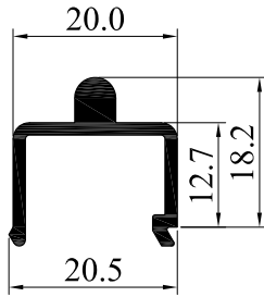
3135-15 0.262 Kg/m
