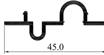
3155-15 0.304 Kg/m
