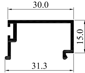
3143-13 0.266 Kg/m
