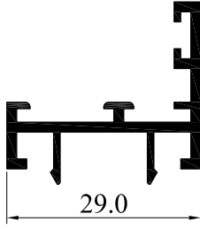
3151-15 0.363 Kg/m
