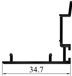
3153-12 0.280 Kg/m
