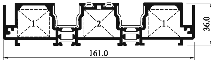
32131-16 ( Üç'lü Üst ve Yan Kasa )
