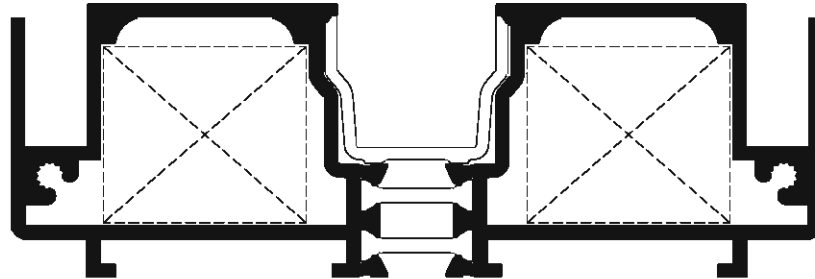
32121-16 Üst ve Yan Kasa ( Gönyeli Kasa )
