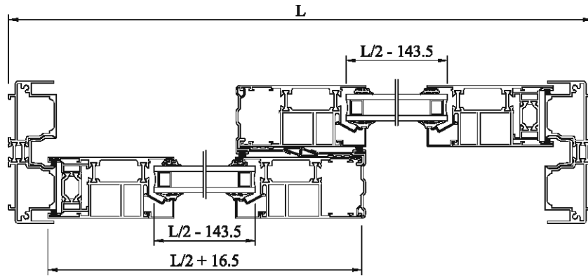
A-A Kesiti
