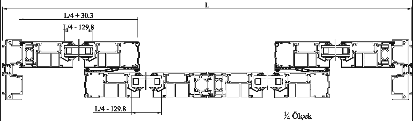
G-G Kesiti
