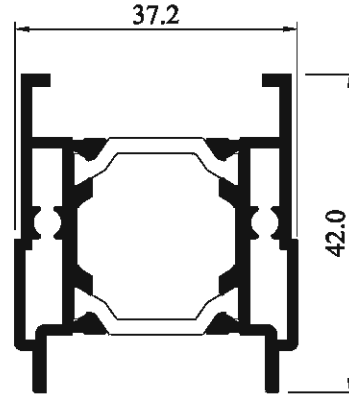
Kanat Birleşim Profili 3215-12
