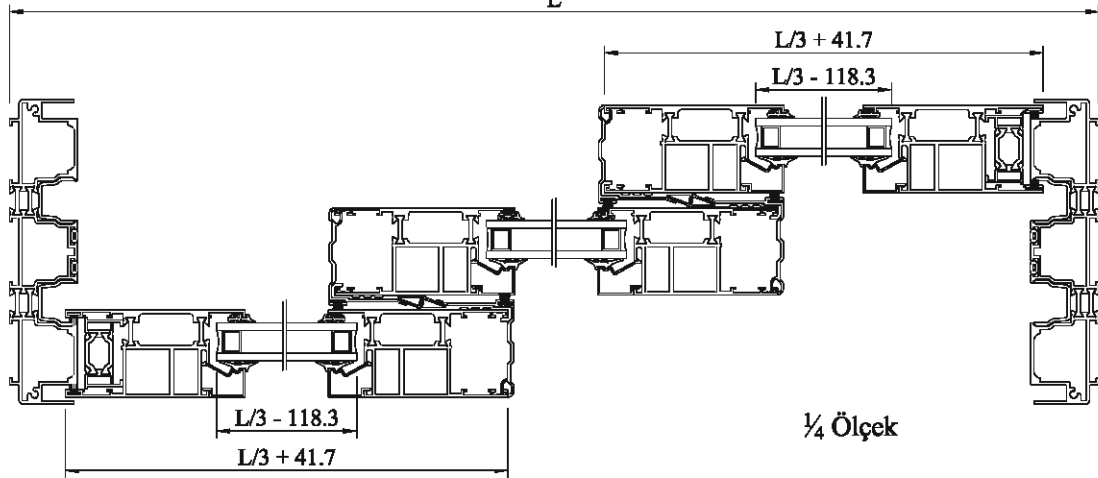
D-D Kesiti L
