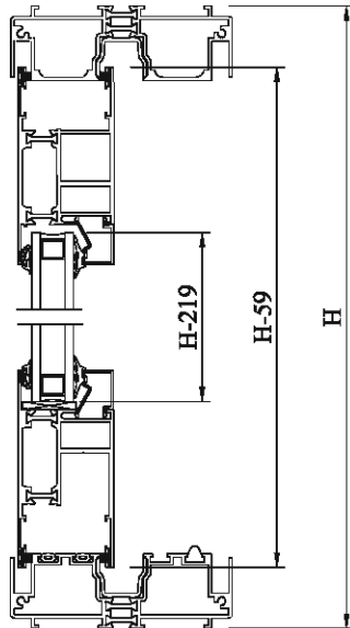
B-B Kesiti
