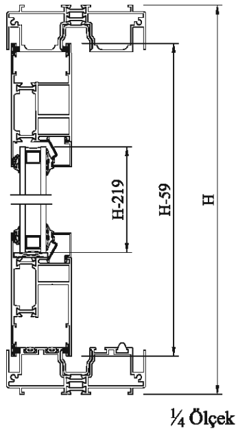
B-B Kesiti
