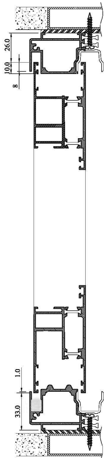
HEBE - SCHIEBE (KALDIR- SÜR) HAREKETLİ KONUM
