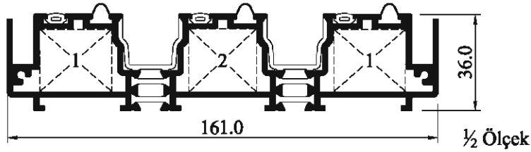
32132-16 ( Üç'lü Alt Kasa )
