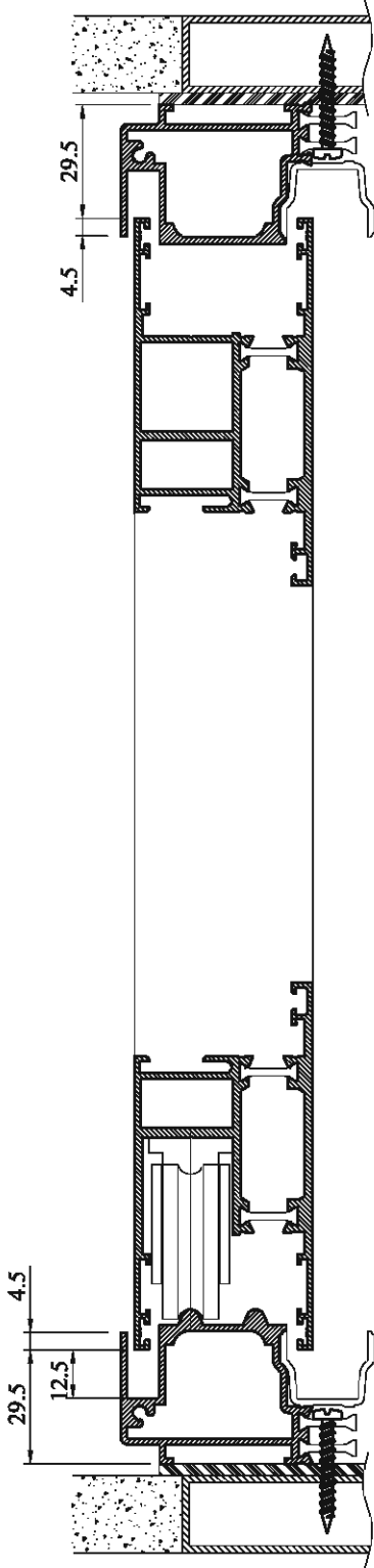
ISI YALITIMLI SÜRME KASA KANAT İLİŞKİSİ (GENÇER RULMANI)
