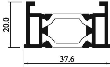
Kilit Adaptör Profili 3219-12
