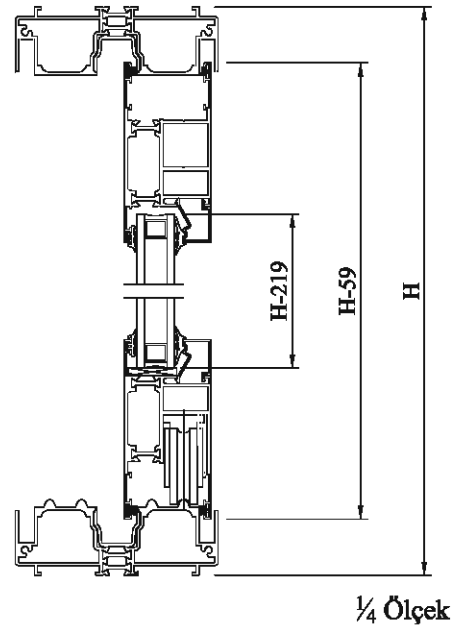
C-C Kesiti
