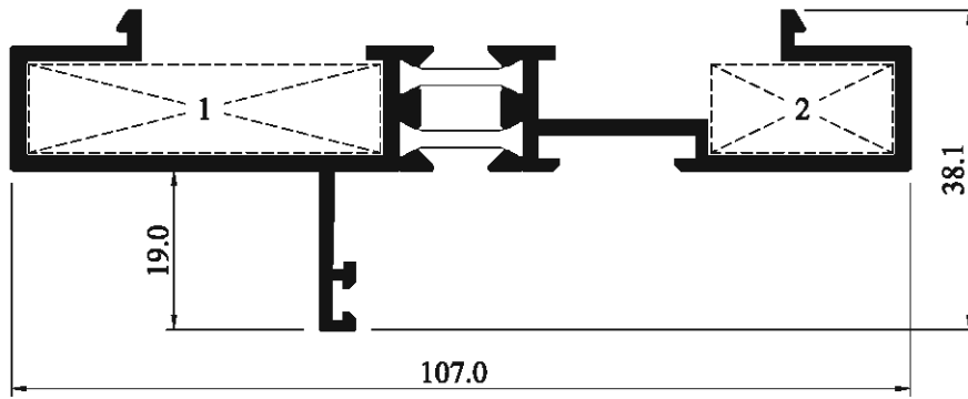
3209-16 Sabit Kasa ( Sabit Cama Geçiş Kasası )
