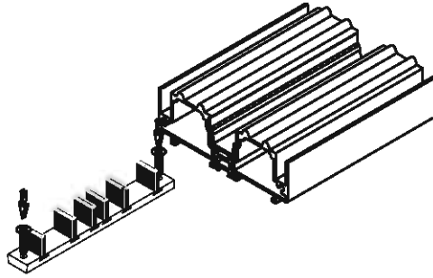
İKİLİ SÜRME KIL FİTİL PLASTİK KULLANIMI
