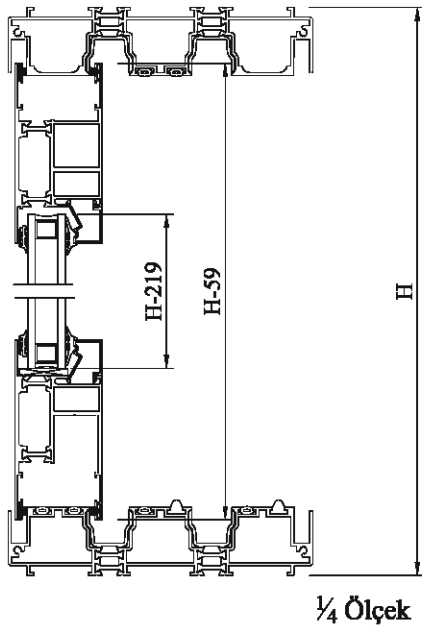
E-E Kesiti
