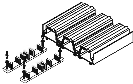
ÜÇLÜ SÜRME KIL FİTİL PLASTİK KULLANIMI
