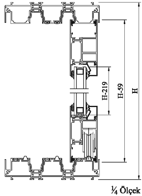
F-F Kesiti
