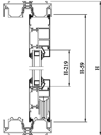
C-C Kesiti
