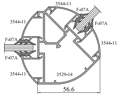
2 Numaralı Detay (45° Açılı Dönüş Detayı)
