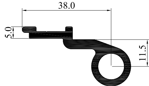
3574-00 Mentşe Profili 0.735 Kg/m
