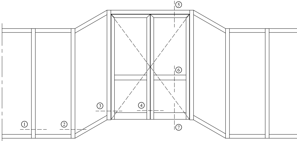
1 Numaralı Detay (Sabit Detayı)
