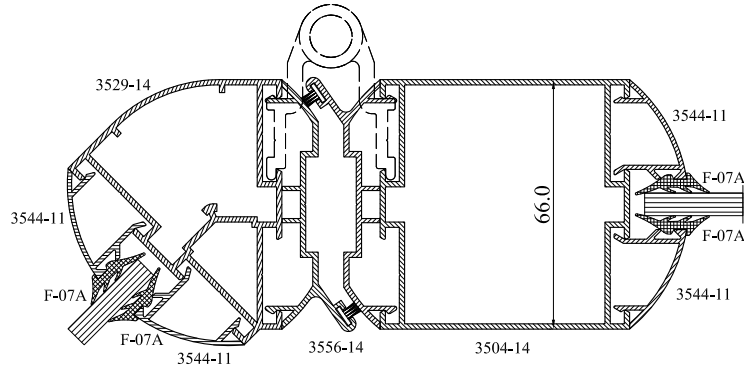
3 Numaralı Detay (45° Açılı Dönüş Sonrası İç Açılır Kapı Menteşe Tarafı) (Çarpma Kapı Menteşesi Takılarak Uygulanabilir)
