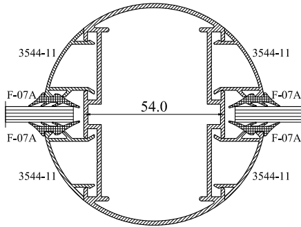
1 Numaralı Detay (Sabit Detayı)
