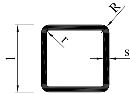
KARE KUTU PROFİLLER RADYÜSLÜ
