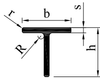
RADYÜSLÜ T PROFİLLER
